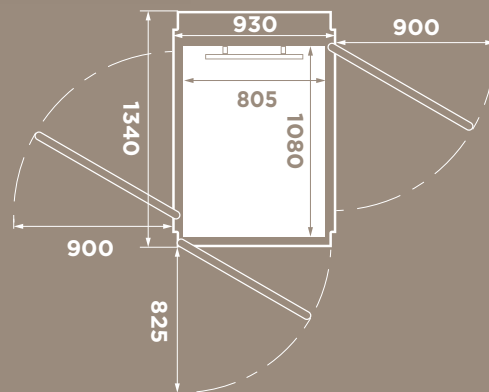
Storlek: 1080 x 805 mm Maxlast: 250 kg / 2 personer
