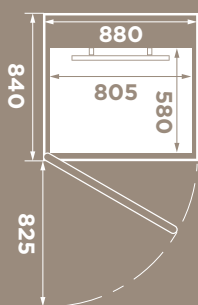
Storlek: 580 x 805 mm Maxlast: 250 kg / 2 personer
